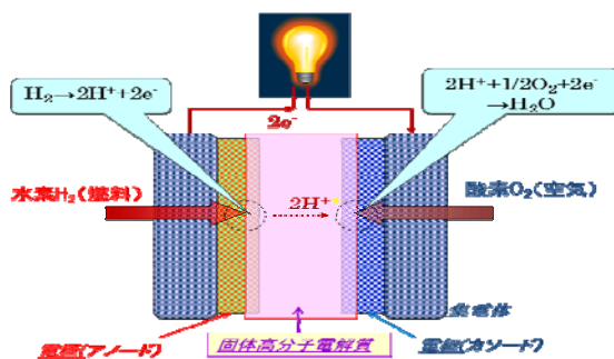
固体高分子形燃料電池のしくみ
