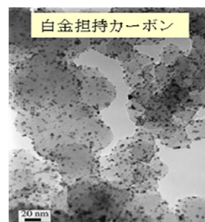
電極触媒のナノ構造(例)
